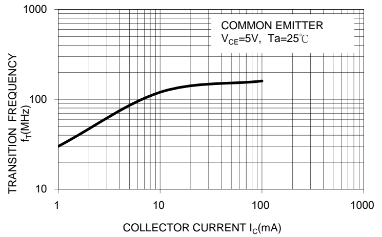
FIG.8 f_T - I_C
